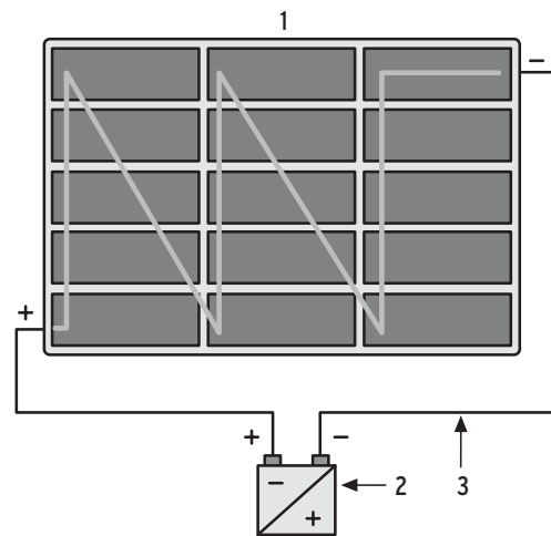
Typischer Systemaufbau:
